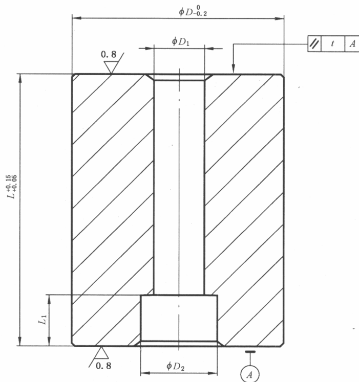
图 2 B型支承柱
