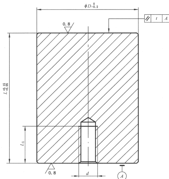
图 1 A 型支承柱
